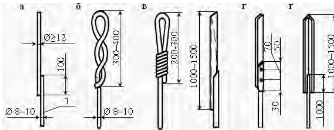
Рис. 14. Конструкції блискавкоприймачів з круглої сталі (а), (б), сталі труби (в), смугової сталі (г), кутової сталі (д): 1 - струмовідвід.
